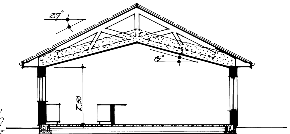
SEKTION, SNITT B-B.
