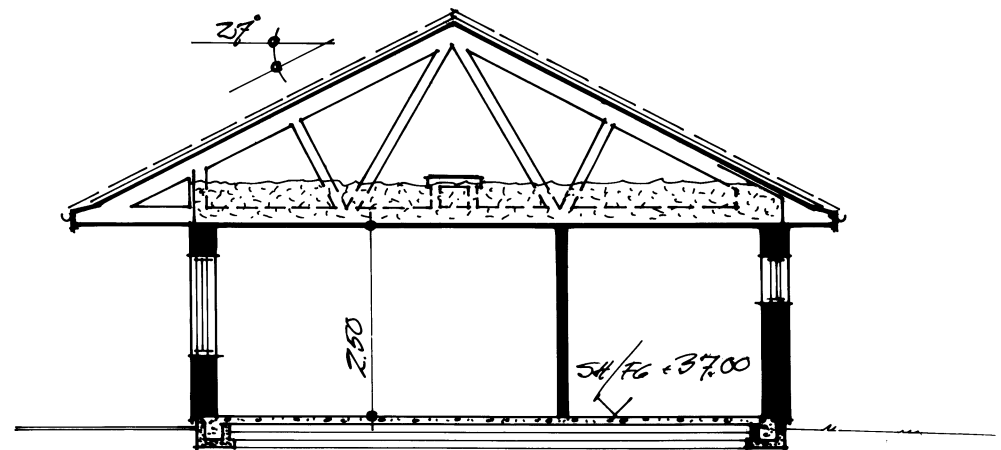
SEKTION, SNITT A-A.
