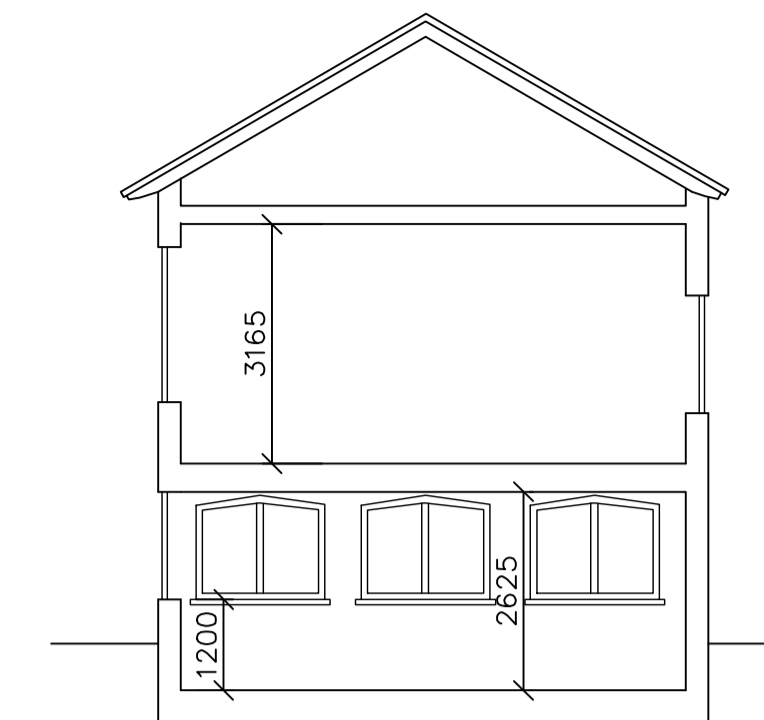
SEKTION A-A
