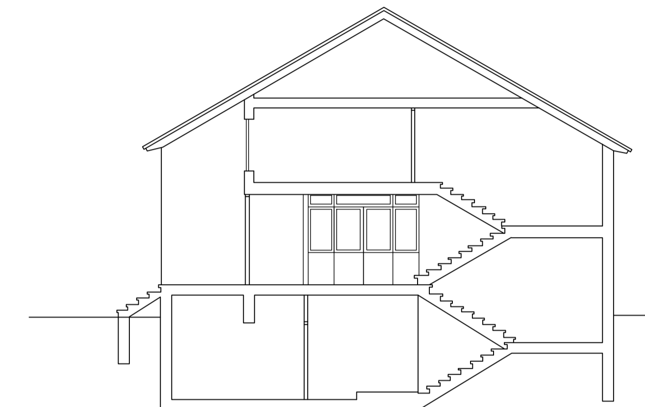
SEKTION B-B
