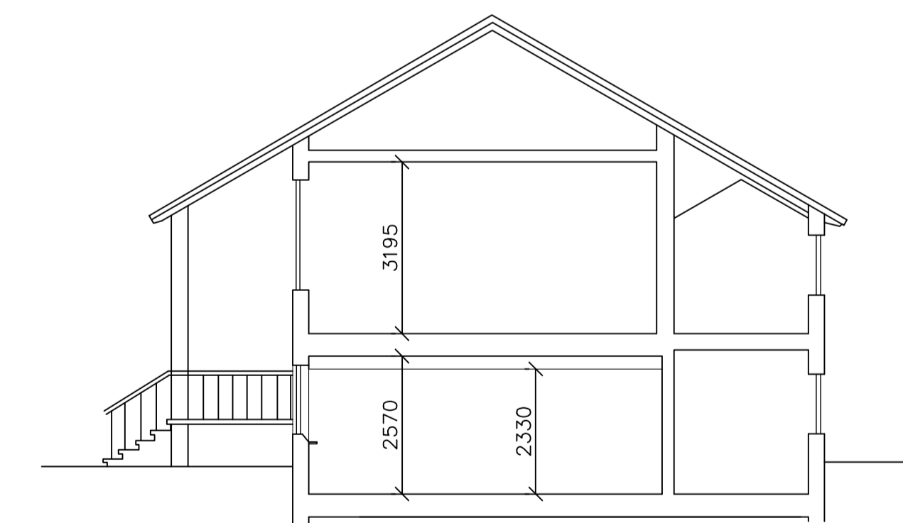
SEKTION C-C
