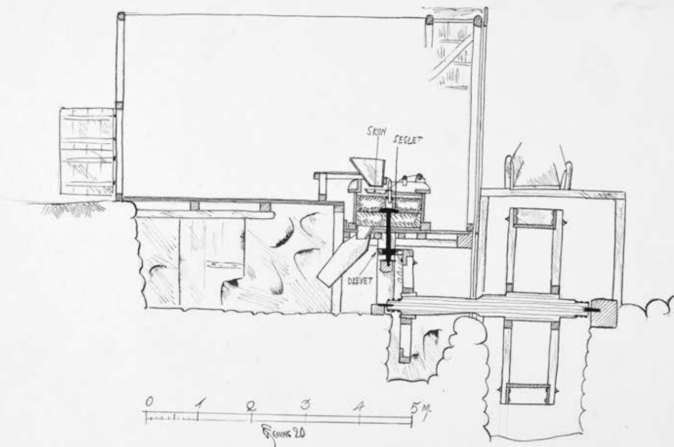
OVANFALLSMÖLLA LÅNGDSEKTION
