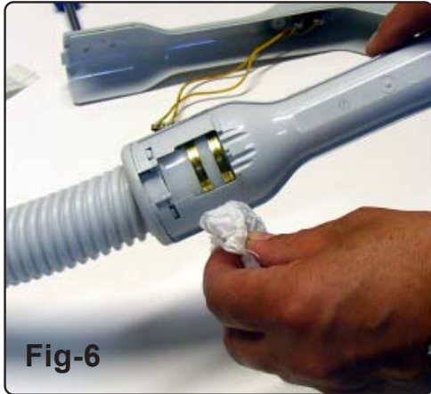
Fig-6. Rengör kontaktytorna noggrant med kemiskt ren bensin eller något liknande.
