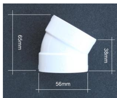
ID-26 Rörböj: Mjuk 30° 2 x Hona.
