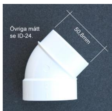
ID-25 Rörböj Spigot: Mjuk 45° böj 1x Hane & Hona.
