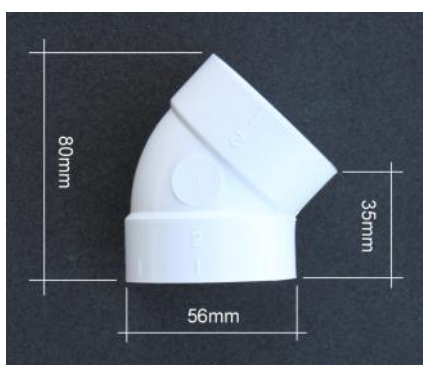
ID-24 Rörböj: Mjuk 45° böj 2 x Hona.
