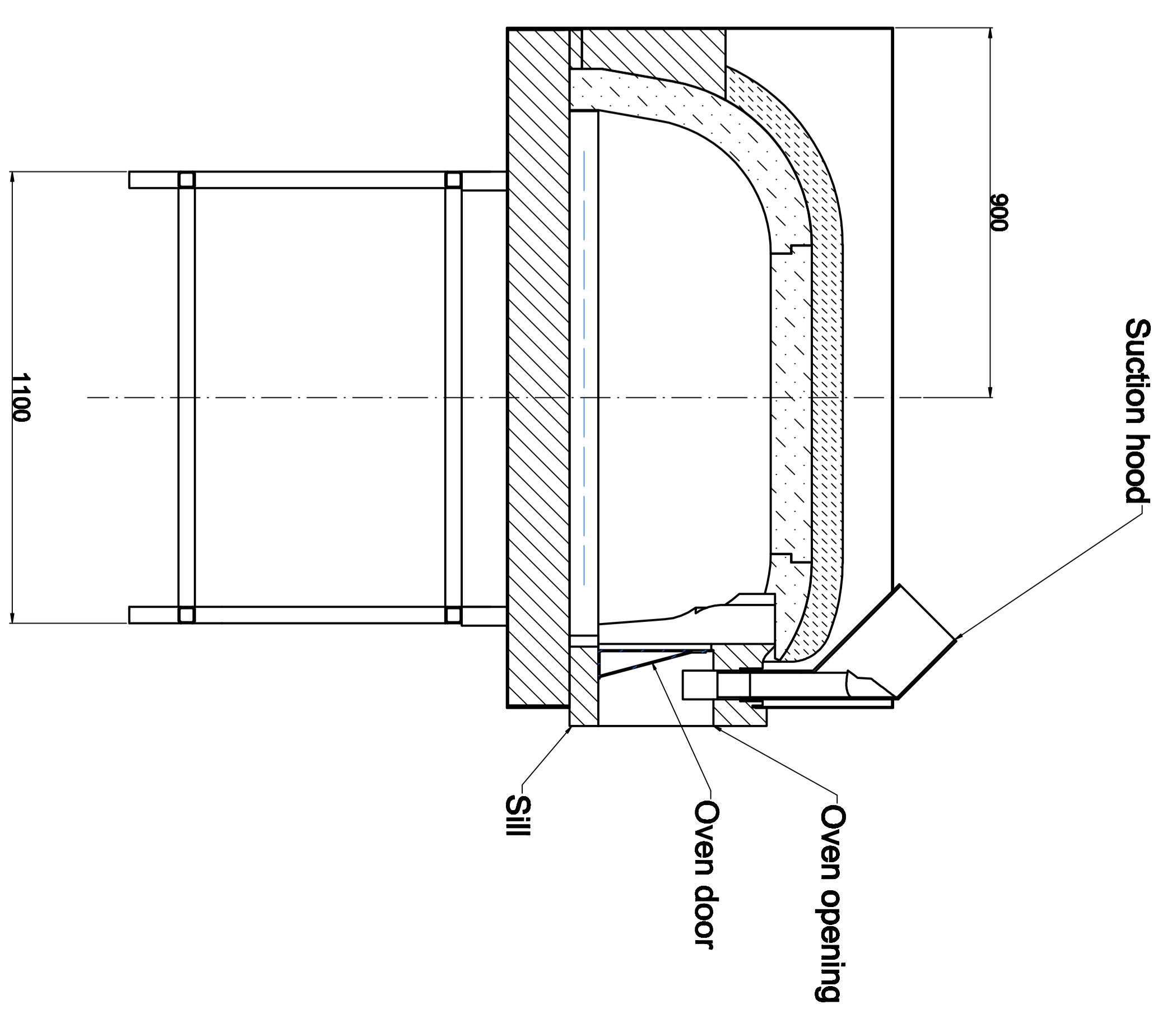
SECTION A-A
