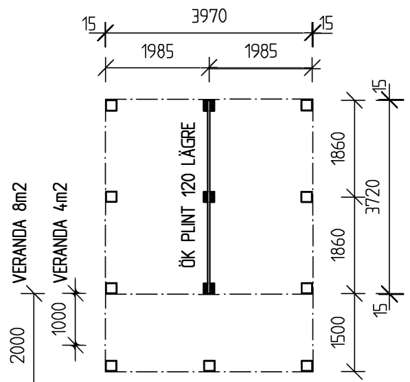
GRUNDPLAN
