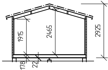
SEKTION
