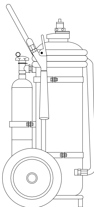
Pulveraggregat med drivgaspatron
