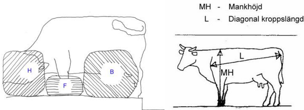
Figur 1. Fria zoner i liggbåset till vänster. Mätning av kroppslängd och mankhöjd till höger. (Kostallplan, 2011).
