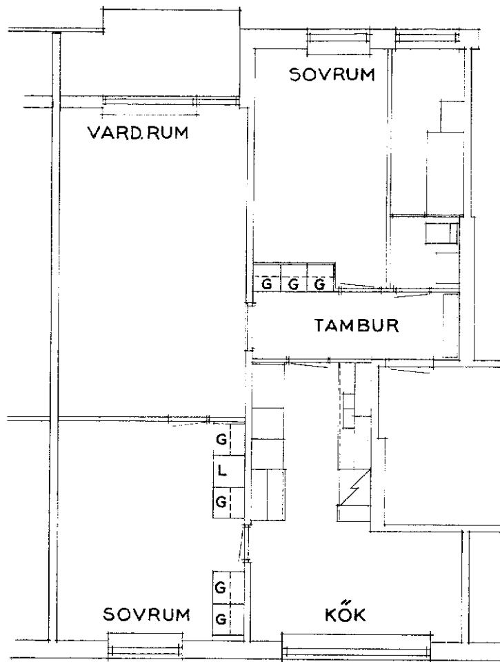
Typ 3 A. 3 rum och kök, 77,8 m 2
