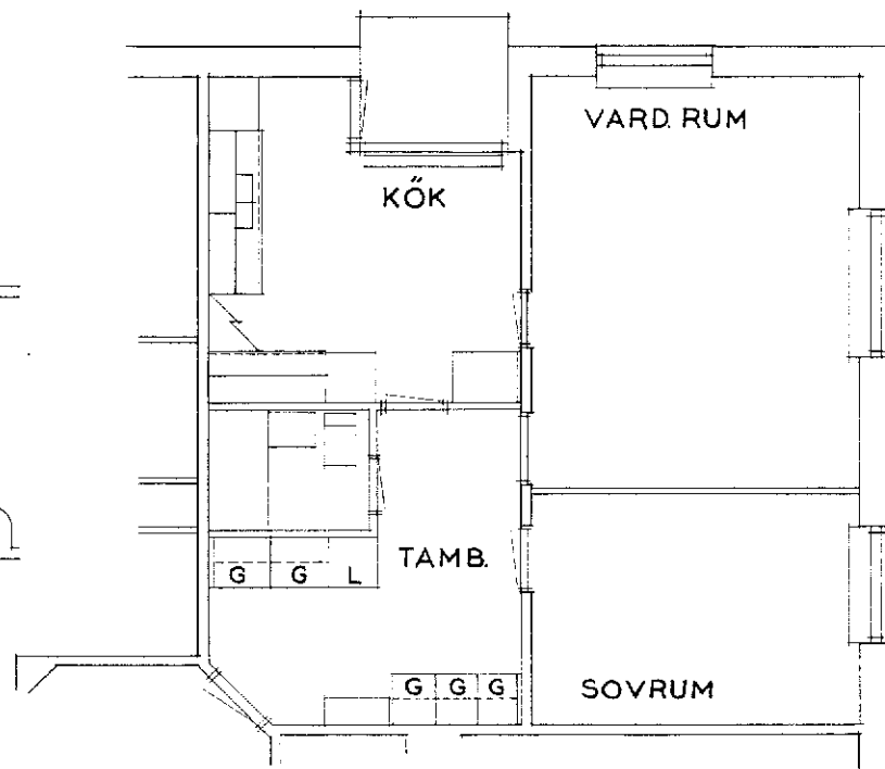
Typ 2 B. 2 rum och kök, 60,3 m 2
