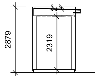
SEKTION FÖRRÅD
