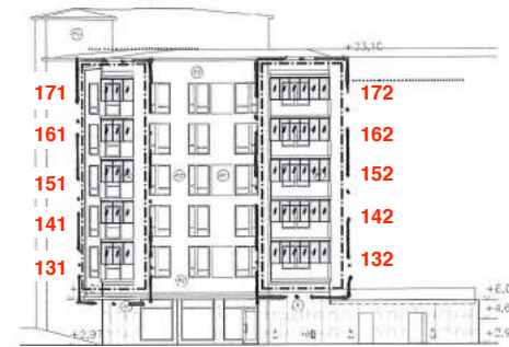
FASAD MOT VÄSTER
