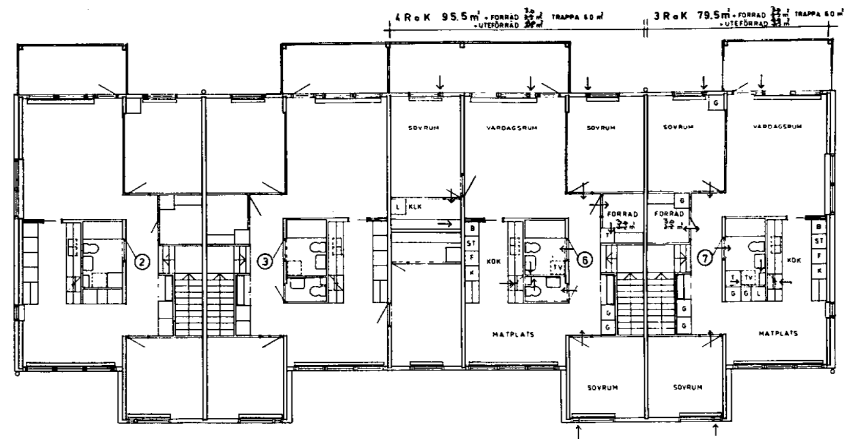
VÄNINGSPÅN 2
