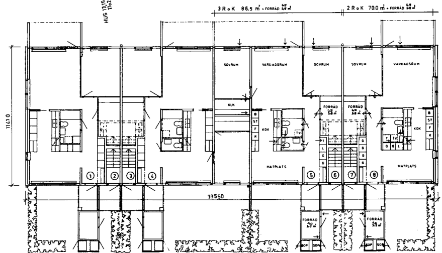
VÄNINGSPÅN 1
