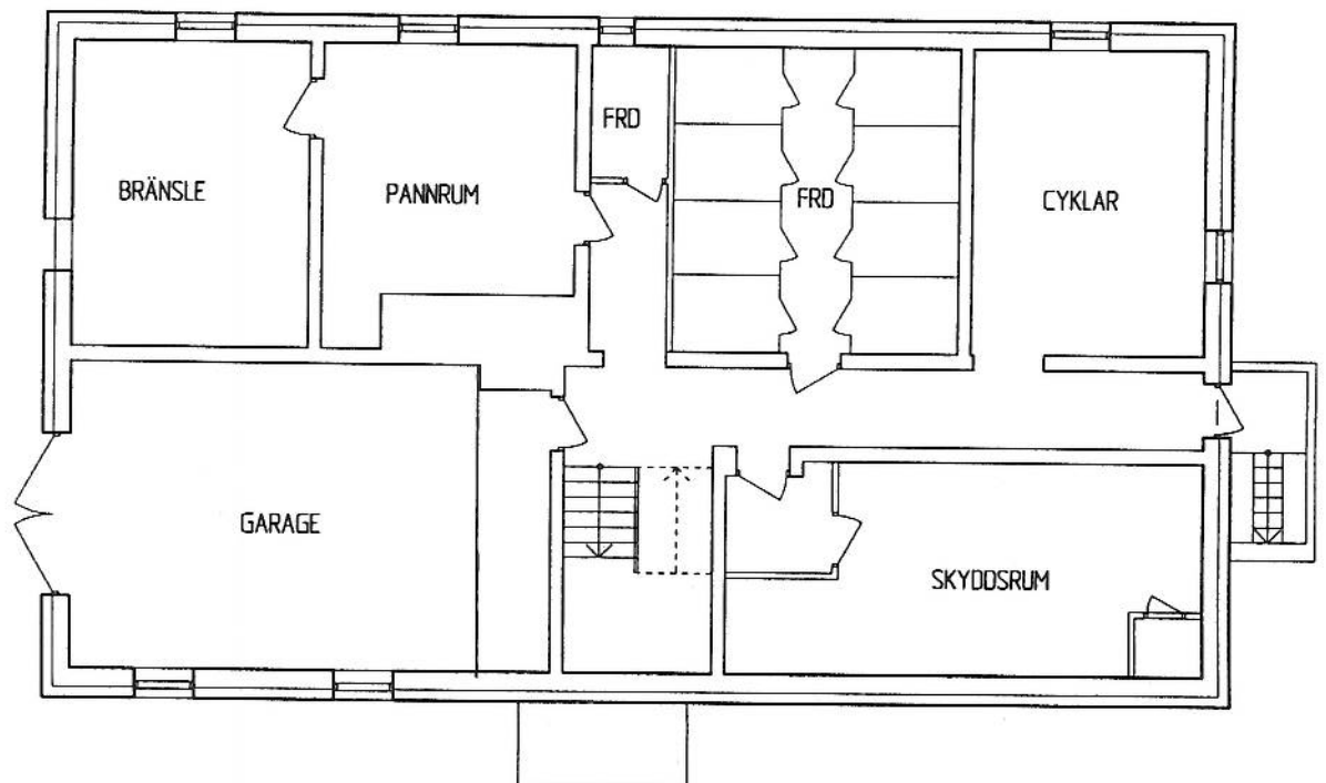
KÄLLARPLAN
